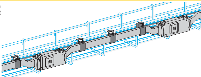
Шинопровод KDP на сетчатом лотке
