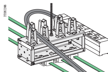
Canalis KDP и VDI в подвесном потолке
