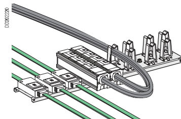
Canalis KDP и VDI в фальшполу
