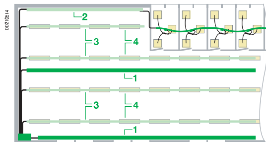
Электрический распределительный щит Prisma Plus G
